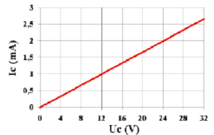
Input : Ic = f( Uc)
